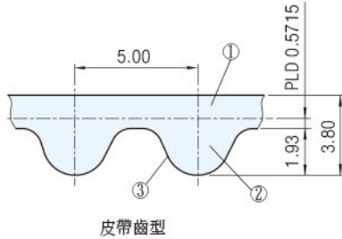
皮帶齒型
