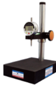
花崗石量測台 GN-MS2015N (不含量表)
