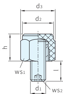
圖 1 公牙
