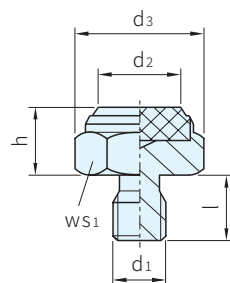
圖 2 公牙
