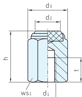
圖 4 母牙
