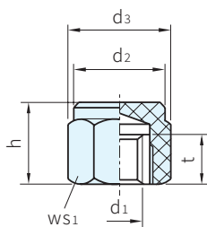
圖 3 母牙
