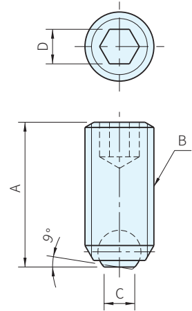
圖 2 平面
