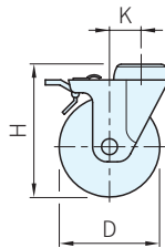
中空剎車輪
