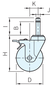
扣環剎車輪
