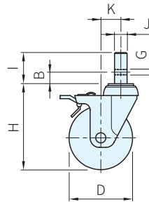
鐵心剎車輪
