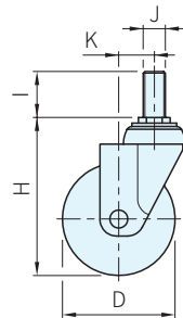
螺絲活動輪
