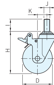
螺絲刹車輪
