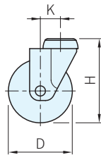
中空活動輪
