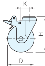
中空剎車輪
