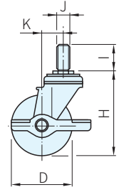
螺絲側剎輪
