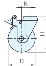
中空剎車輪
