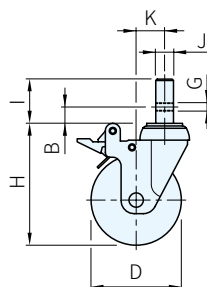
鐵心剎車輪
