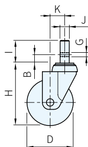
鐵心活動輪
