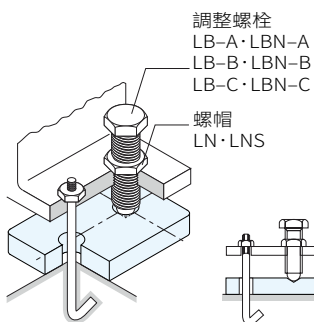
微調機械的水平簡單
