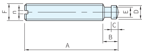
一字溝
