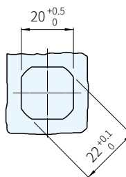
開孔尺寸
