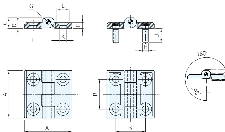
圖1 (鎖固型)
