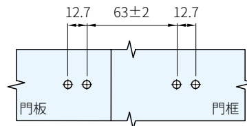
開孔尺寸
