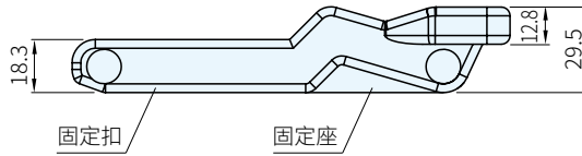
固定扣
