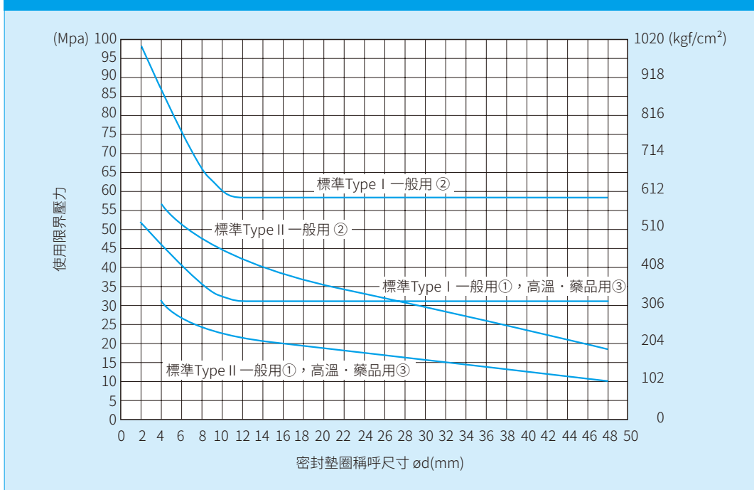
圖2 靜態使用限界壓力
