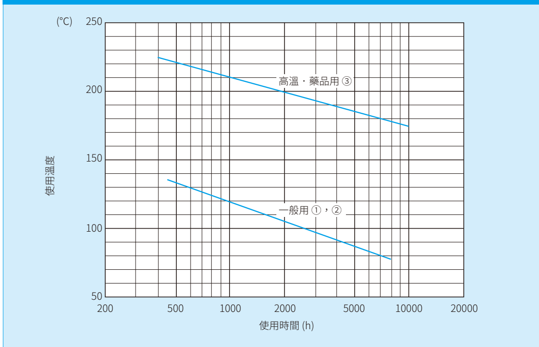
圖1 溫度與時間的關係
