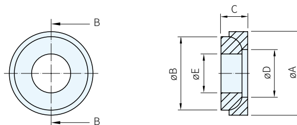
B-B剖面
