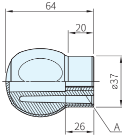
母牙 EBK-SOFT
