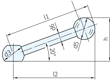
手鈕 DIN 319
