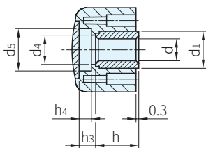
剖面 X-X
