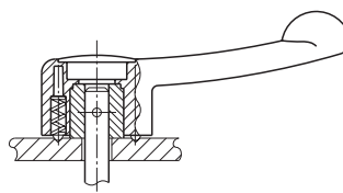
⑥卡扣式
