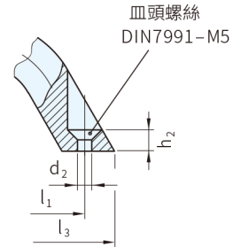
圖2 (外裝型)
