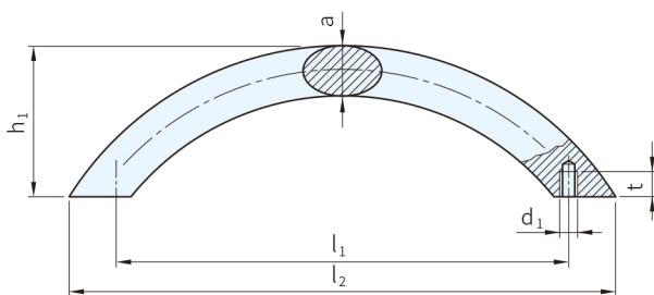
圖1 (內裝型)
