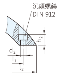
圖2 (外裝型)
