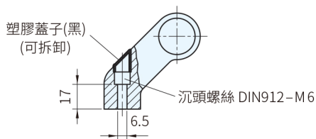
圖2 (外裝型)
