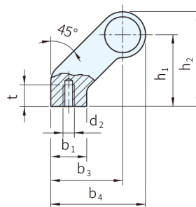
圖1 (內裝型)
