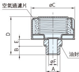
SMN (排氣型)
