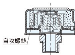
SMW (壓力型)
