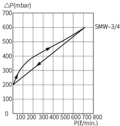
SMW(壓力型)
