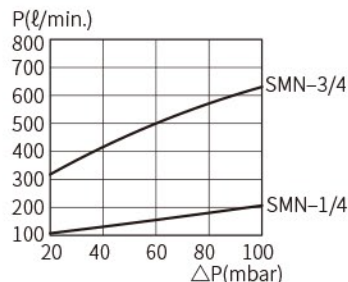
SMN(排氣型)
