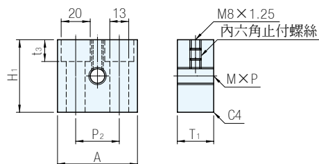
④ 固定板
