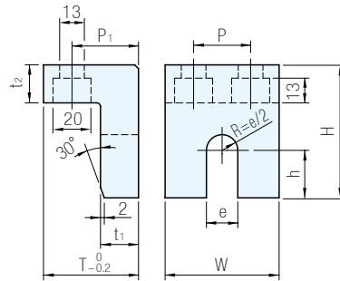
⑤ 支持座
