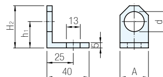
⑤ 支持座
