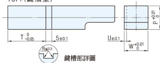
TSPF(鍵槽型)
