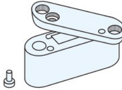
② 以彈簧銷為支點,旋轉墊板,就可以簡單的更換日期的下一位(也可拆下墊板)
