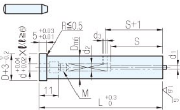
基本型定位銷孔頂料型冲頭 PIT-E、PIXT-E、PIT-E、PIXT-E
