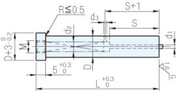
基本頂料型冲頭
