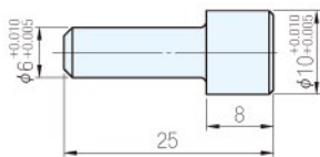
D38、45用定位銷 PIT-ENP
