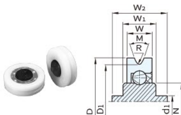
圖 5(孔型)
