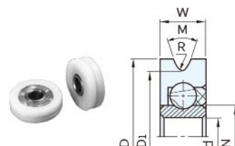
圖 3(孔型)
