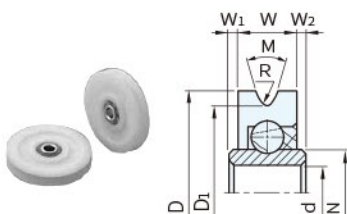
圖 4(孔型)
