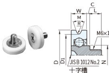
圖 2(螺栓)
