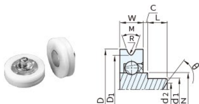
圖 1(鉚合)
