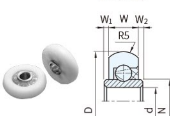
圖 5(孔型)
