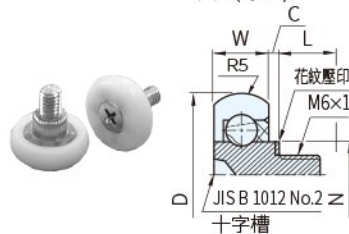
圖 3(螺柱)
