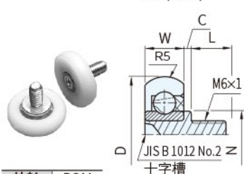
圖 4(螺柱)
