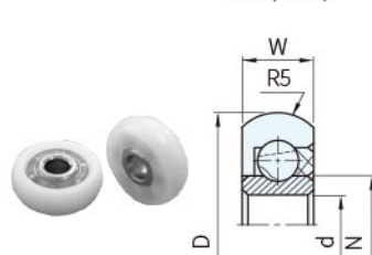
圖 6(孔型)
