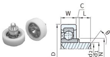
圖 1(鉚合)
