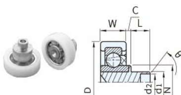
圖 2(鉚合)
