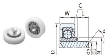
圖 3(鉚合)
