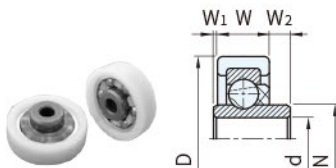
圖 5(孔型)
