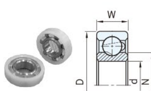
圖19(孔型)
