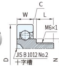
圖16(螺栓型)
