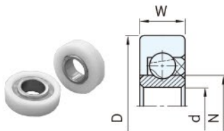
圖18(孔型)
