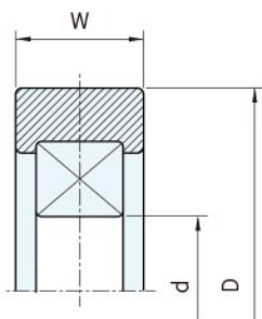
圖 1(孔型)
