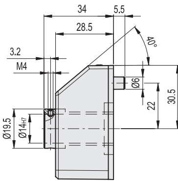
DD51-E-RF-SST-IP65
