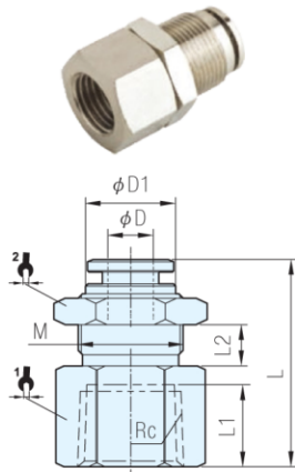
MPMF 全銅隔板內螺紋直通
