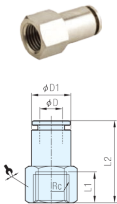
MPCF 全銅內螺紋直通
