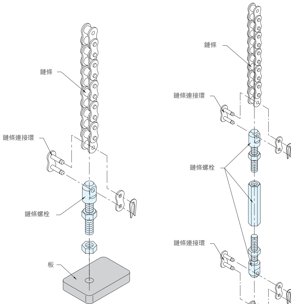
平衡塊的鏈條固定簡單
