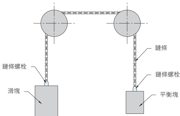
平衡塊的鏈條固定簡單
