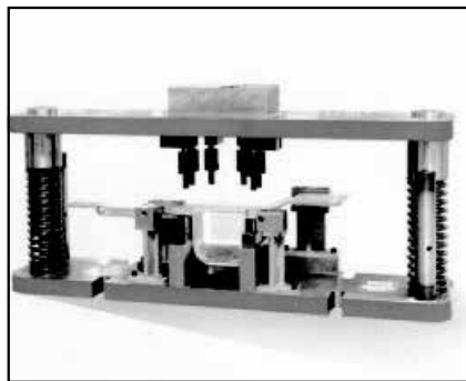
Tog-L-Loc 使用於鋁合金汽車零件壓合
