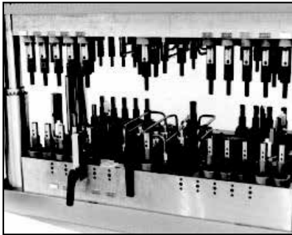
Tog-L-Loc 使用於暖氣爐壓合
