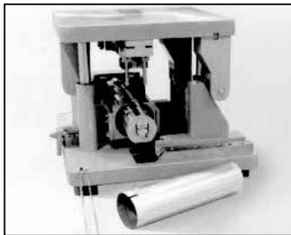
Tog-L-Loc 使用於排氣管壓合
