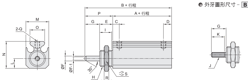
● 外牙圖形尺寸 - B
