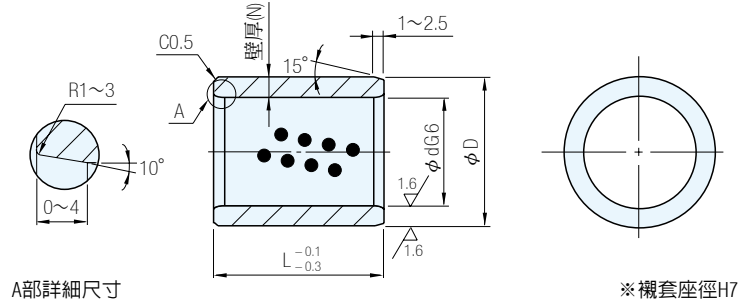
A部詳細尺寸
