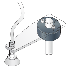
板的安裝
