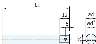
TRA-B (實心)
