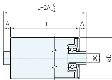
TRA D=32,38,42,60,76
