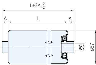
TRA D=57
