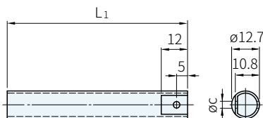
TRA-A (空心)
