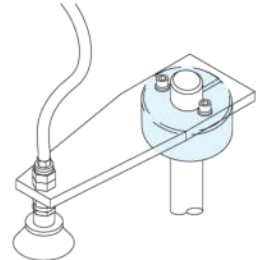
SCS 螺牙孔型 平板安裝
