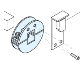
角軸用 感應器支架安裝
