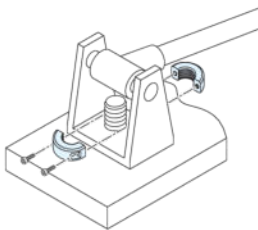
SCSS 內徑螺牙型 螺桿軸固定
