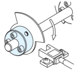
SC 3孔固定環 限位器安裝
