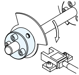
SC 3孔固定環 限位器安裝
