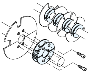
圓軸用 限位器安裝
