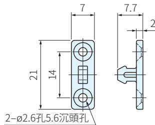
PR4PK-1 (木製品用門門NO.1) 訂購品
