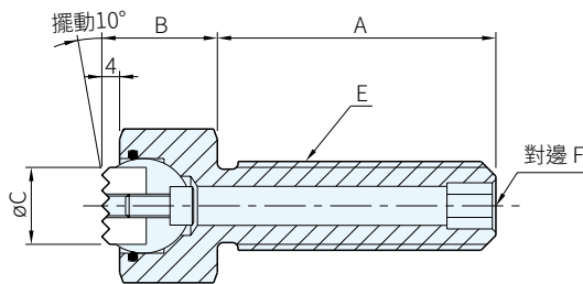
BUH-S 10015~24100 (齒面)
