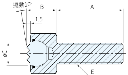
BUH-S 06012~08040 (齒面)
