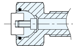
BUH-F 10015~24100 (平面) BUH-E 10015~24100 (POM塑膠)
