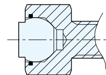
BUH-F 06012~08040 (平面) BUH-E 06012~08040 (POM塑膠)
