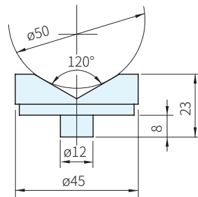
V型蓋
