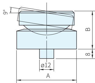
自調型蓋
