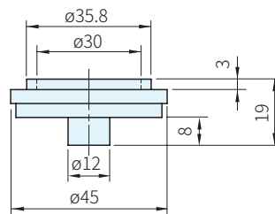
盤型蓋
