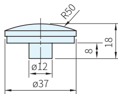
球狀型蓋
