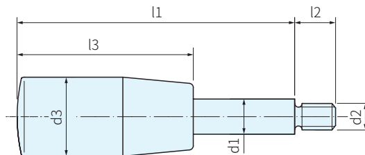
圖2 (圓柱型手柄)
