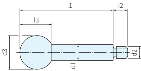
圖1 (球型手柄)
