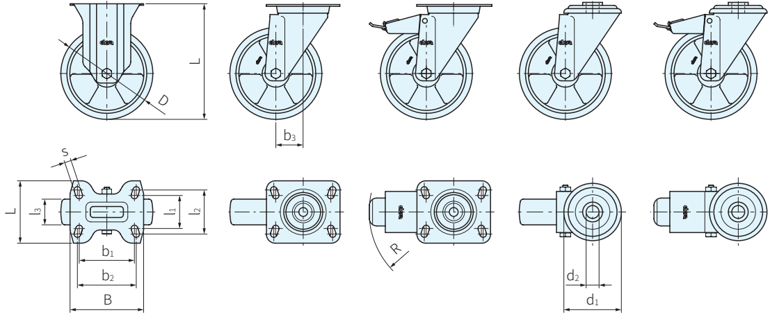
RE.F5-PSL-N 固定輪
