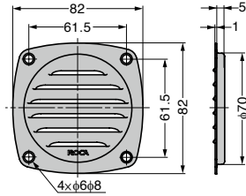
Ventilator body
