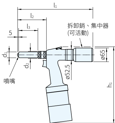
圖1 — 氣動式
