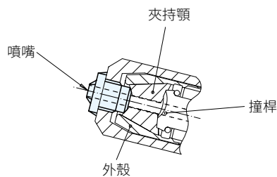
圖2 — 維修零件
